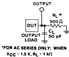
Fig. 4 - Test circuit.
