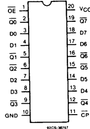
CD54/74AC/ACT534
