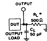
Fig. 5 - Test circuit.
