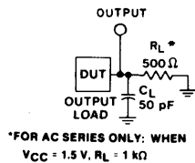
Fig. 6 - Test circuit.
