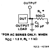
Fig. 5 - Test circuit.
